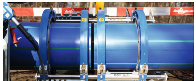
Zuverlässiges Schweißen mit der Stumpfschweissmaschine Top 2.0 630 für eine langhaltende Verbindung.
